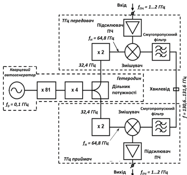
Рис. 9. Структурна схема дослідного зразка прийомопередавача ТГц діапазону
