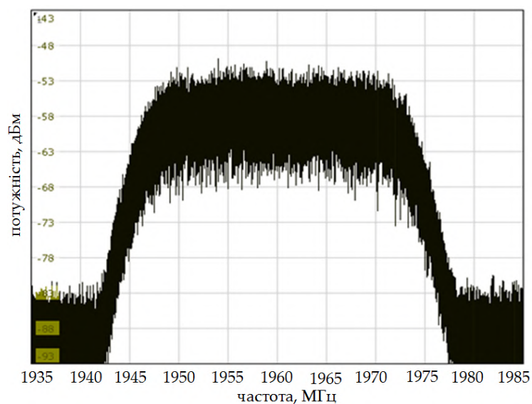
Рис. 12. Результати дослідження спектру сигналу DVB-S на частоті 1,96 ГГц на виході приймача терагерцового діапазону
